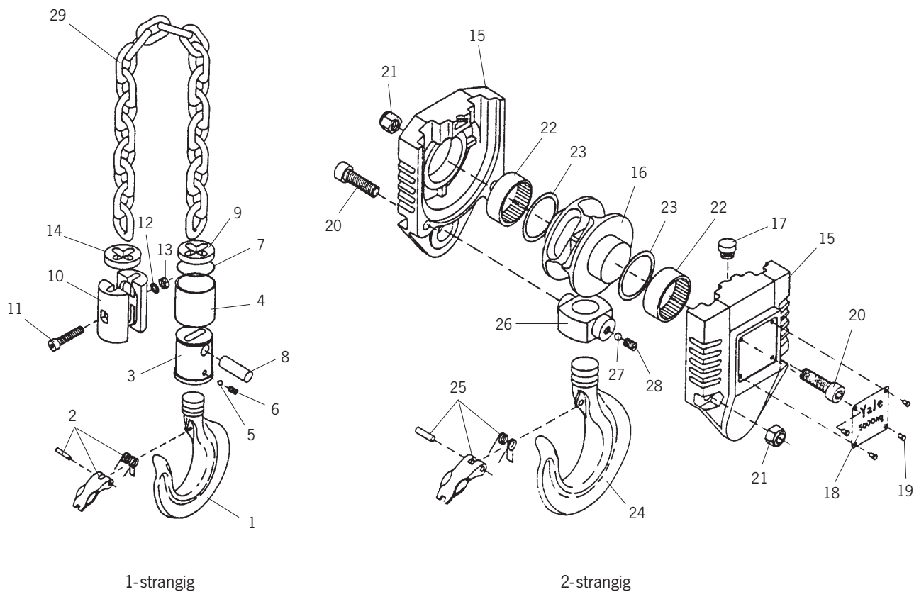
Fig. 21: Unterflaschen (CPE/F 1.600 - 5.000kg)
