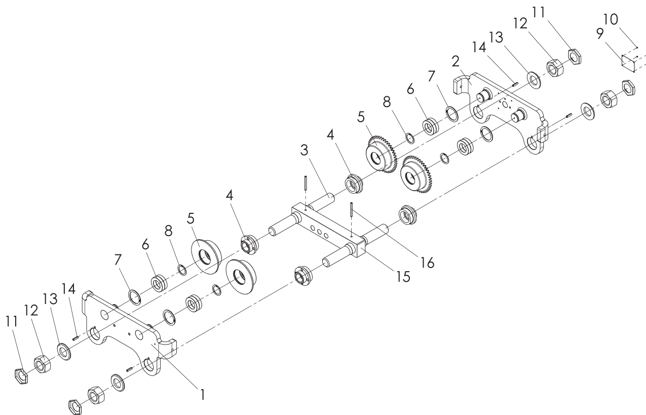
Fig. 31: Rollfahrwerk
