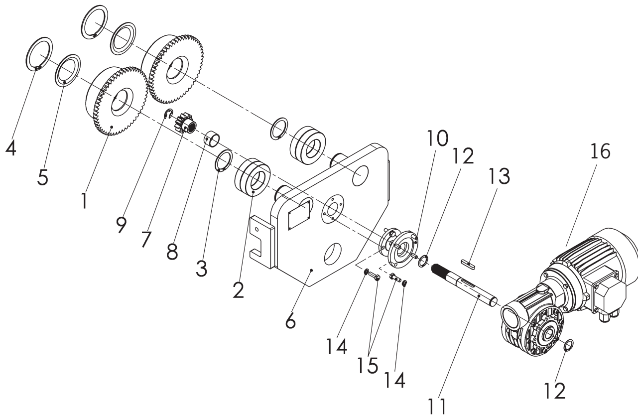
Fig. 35: Elektroantrieb für Fahrwerk CPE/F 7.500 - 10.000kg (übrige Teile siehe Rollfahrwerk)
